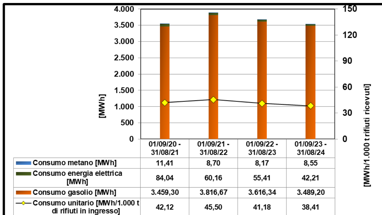
Grafico 6.4 Consumo energetico totale
