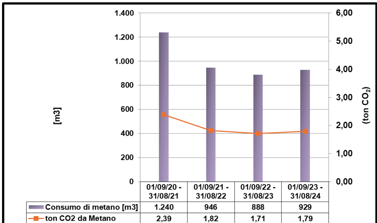
Grafico 6.3 Consumo di combustibile per riscaldamento
